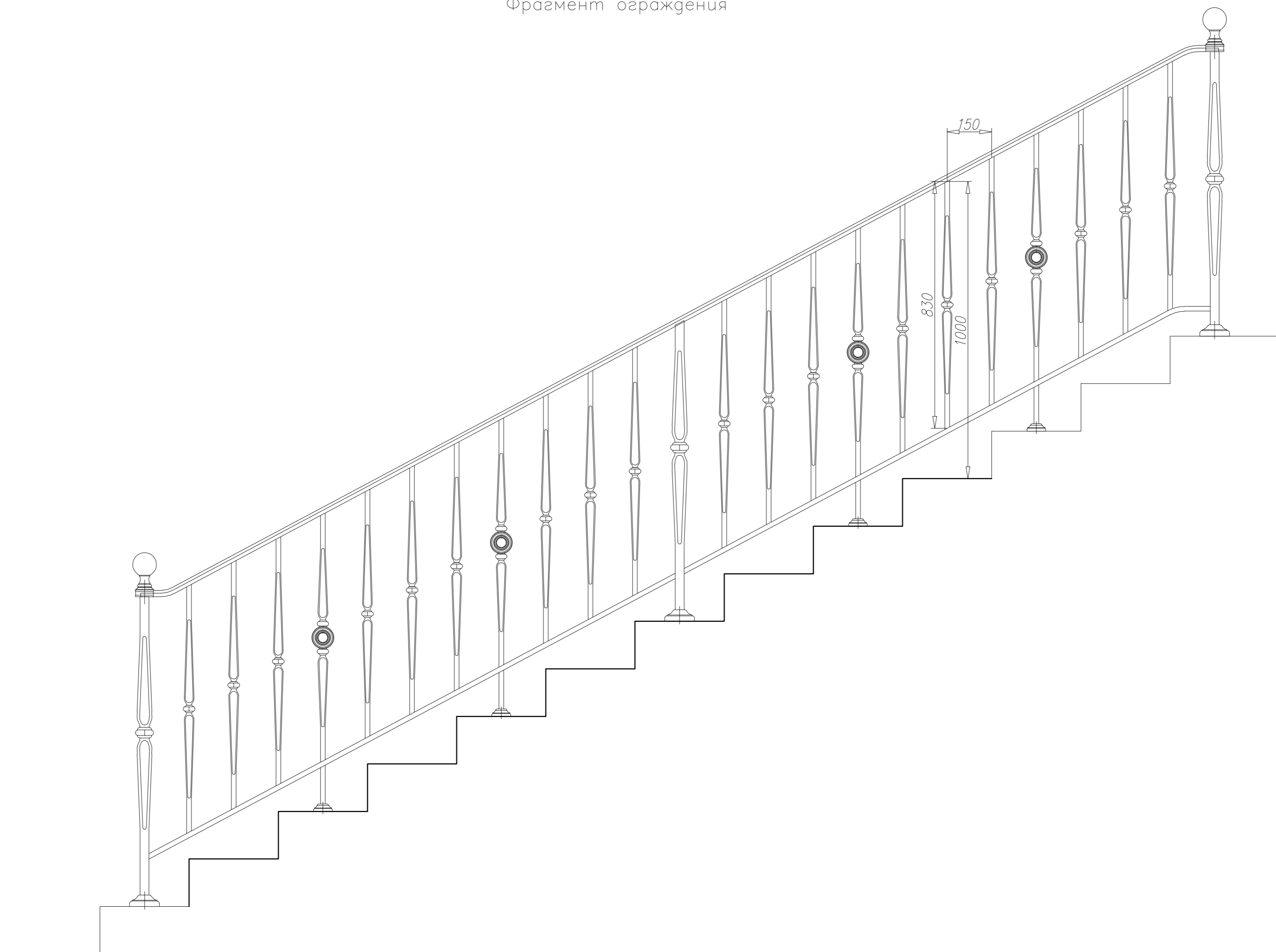
Серия "Рондо" Вариант 10 Фрагмент ограждения
